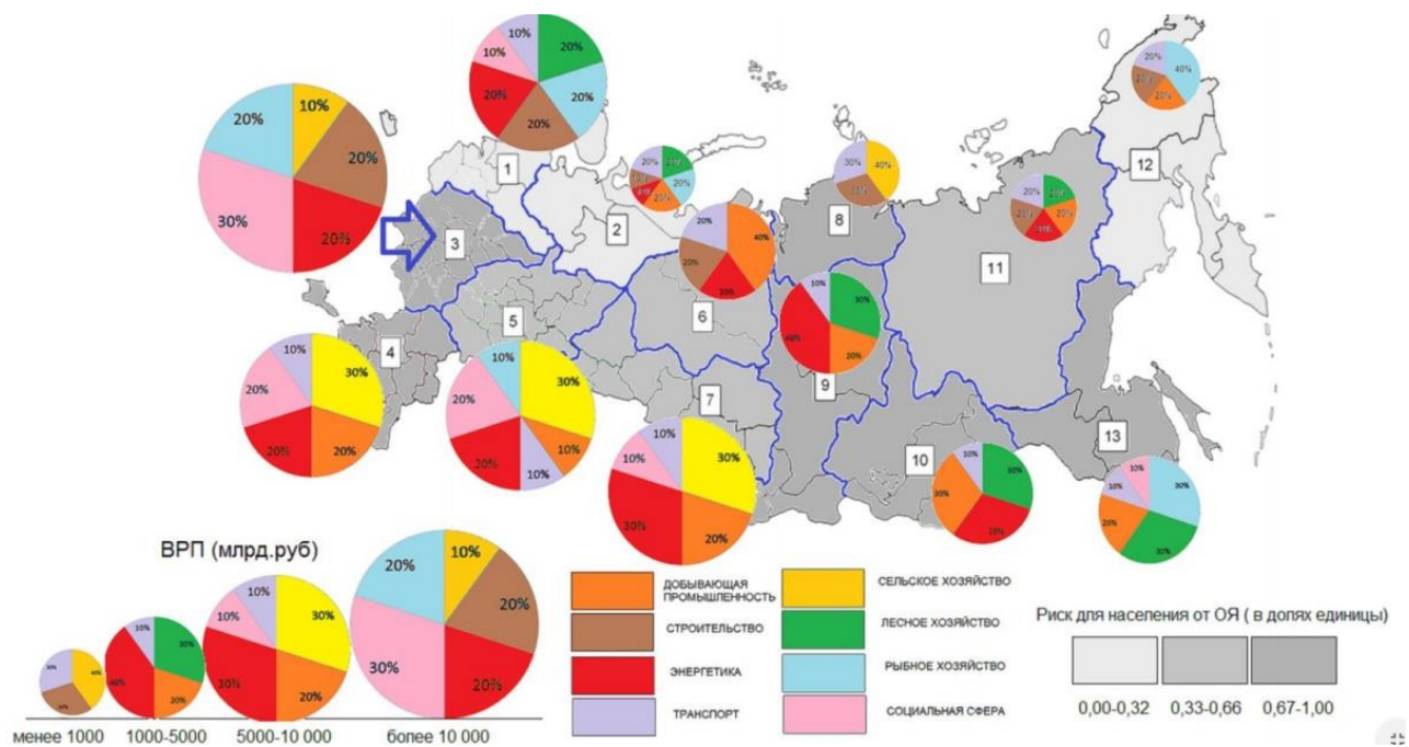
Прогноз индекса геоэкологических рисков на середину XXI в. Расчет проведен с использованием оптимизированной климатической перспективной оценки по ансамблю моделей CMIP5.
