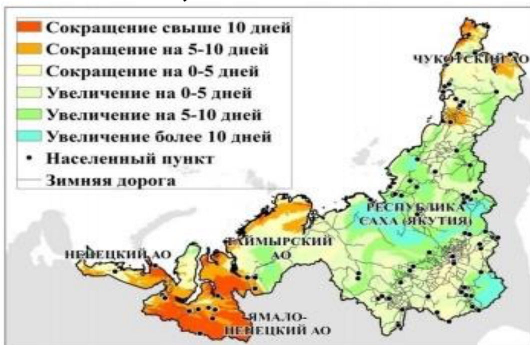
Изменения расчетной продолжительности эксплуатации зимних дорог в период между 1965–1975 и 1995–2005 гг.
