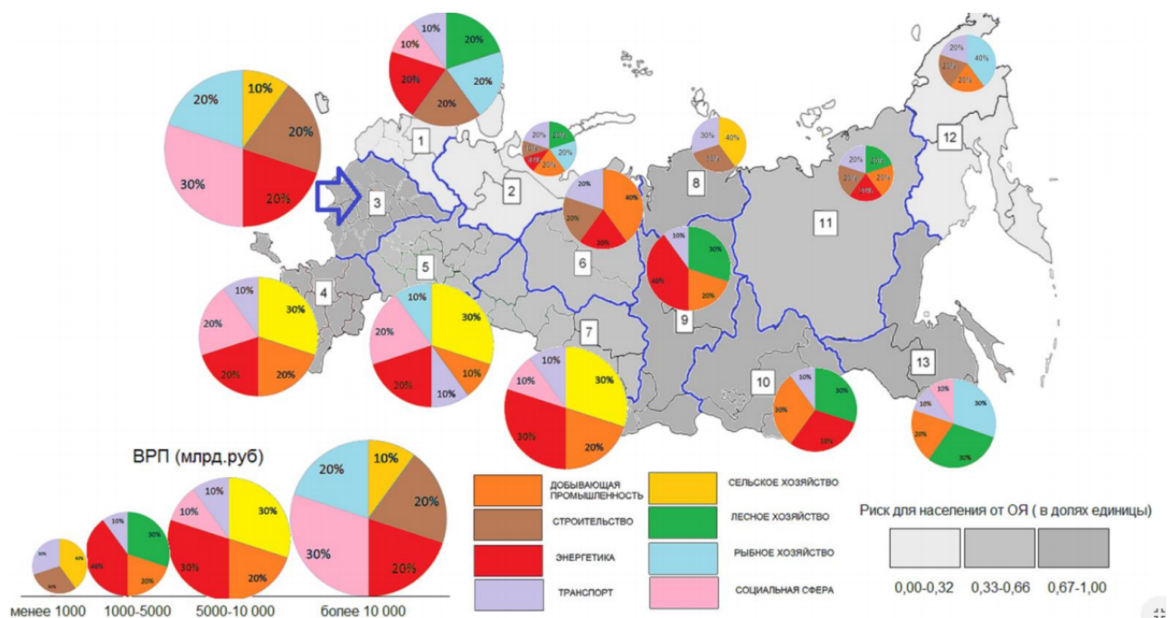
Прогноз индекса геоэкологических рисков на середину XXI в. Расчет проведен с использованием оптимизированной климатической перспективной оценки по ансамблю моделей СМIP5.
