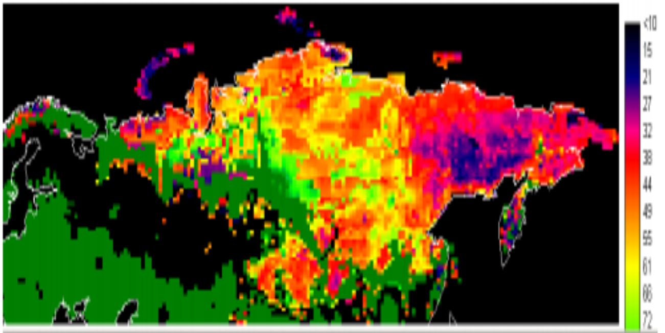
Прогноз индекса геоэкологических рисков на середину XXI в. Расчет проведен с использованием оптимизированной климатической перспективной оценки по ансамблю моделей СМIP5.
