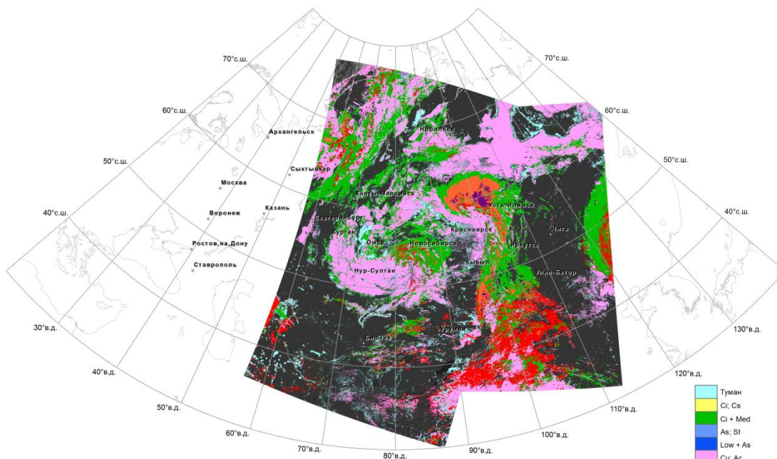
Монтаж космических изображений. Типы облачности.
