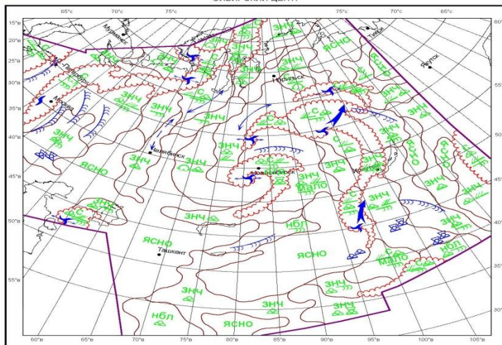
КАРТА НЕФАНАЛИЗА И ПРОГНОЗА ЭВОЛЮЦИИ ОБЛАЧНЫХ ОБРАЗОВАНИЙ
