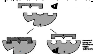
S - субстрат, E - фермент, I - ингибитор
