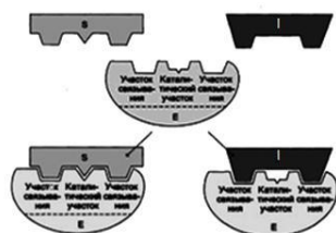
S - субстрат, E - фермент, I - ингибитор
